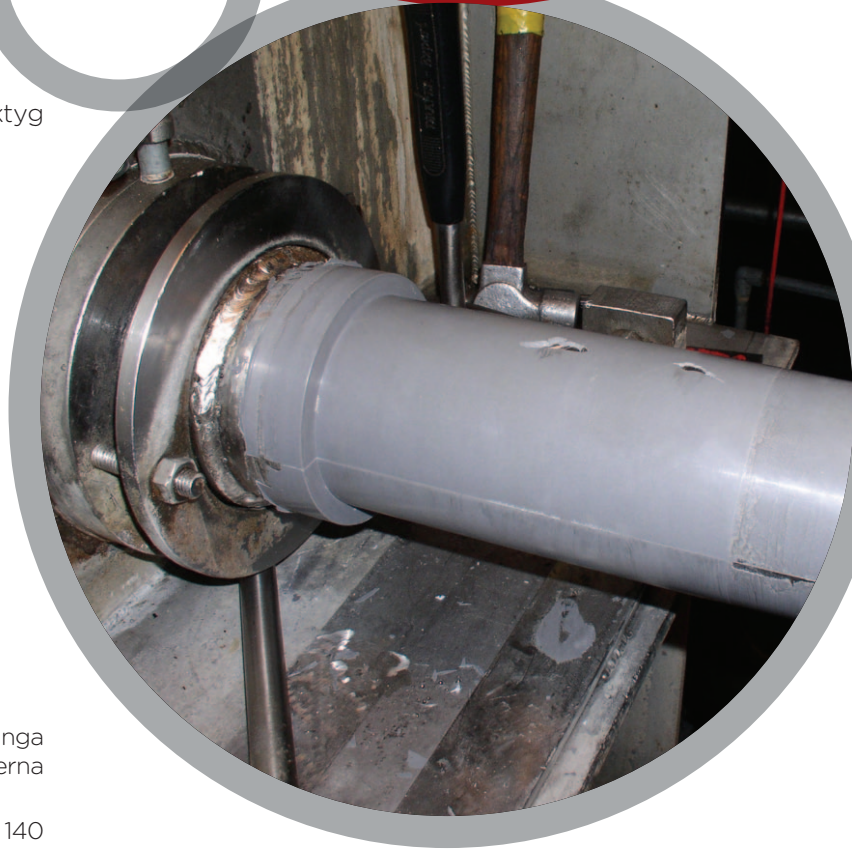
Axelreparation
